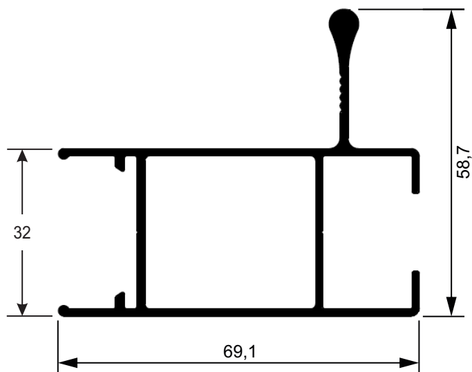
AK327 Montante lateral e central 5,77 Kg/Br
