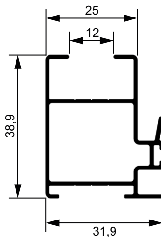
90056 Montante mão amiga 3,26 Kg/Br interno e externo
