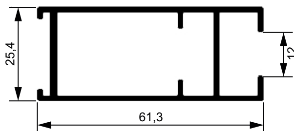
SK241 Montante da folha sem baguete 4,20 Kg/Br
