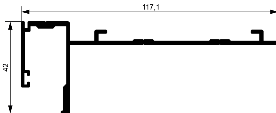
NG101 Perfil suporte inferior para corrimão Neograd 5,93 Kg/Br
