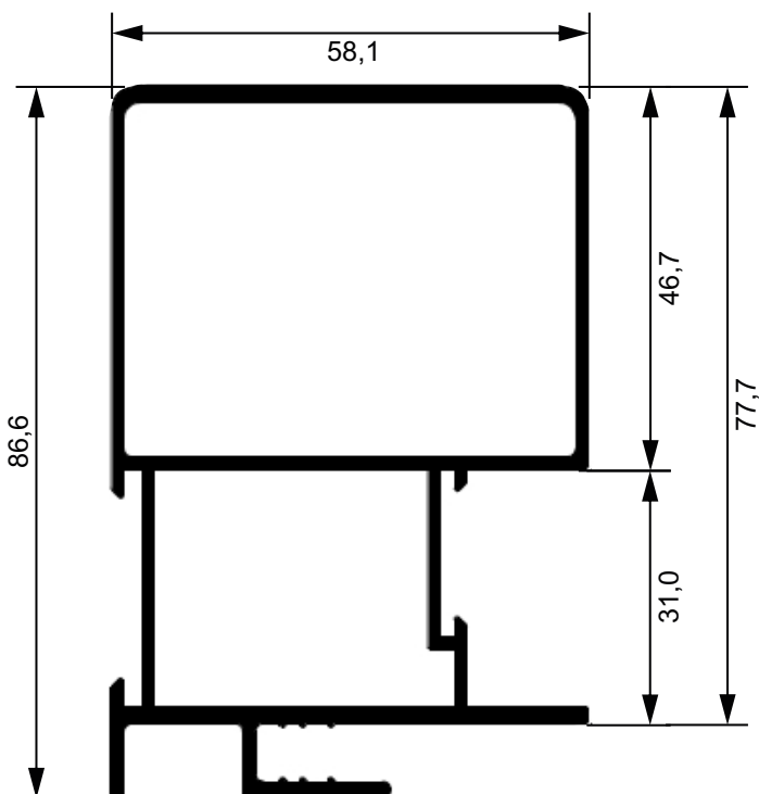
AK512 Montante mão amiga tubular. Linha Aglo 3.2 8,37 Kg/Br 5000
