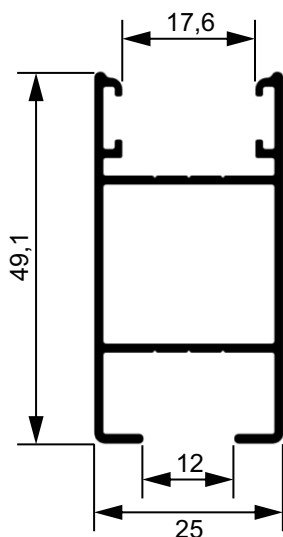
90055 Montante lateral 3,26 Kg/Br
