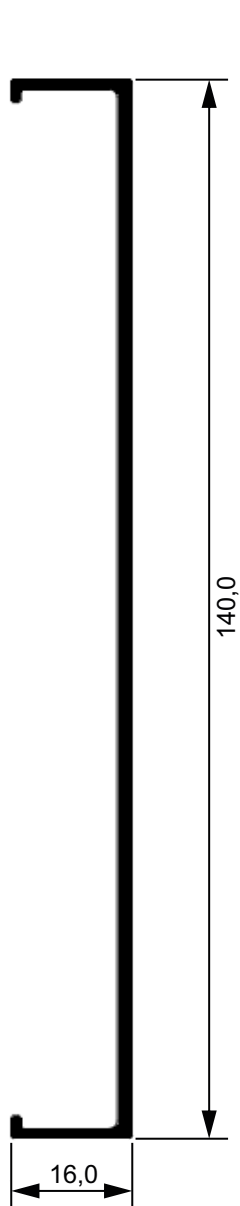
AK243 Marco lateral 5,22 Kg/Br Linha Aglo 2.0
