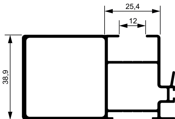
90061 Montante mão amiga tubular 6,38 Kg/Br
