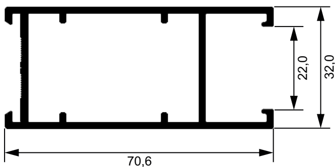
AK509 Travessa inferior e superior. 6,15 Kg/Br Linha Aglo 3.2
