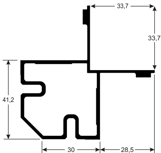
UF095 Coluna vertical de canto aberta - 36mm 8,35 Kg/Br
