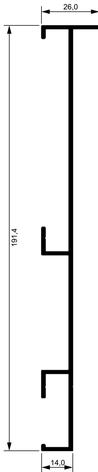
AK507 Marco lateral 4 planos 8,14 Kg/Br Linha Aglo 3.2
