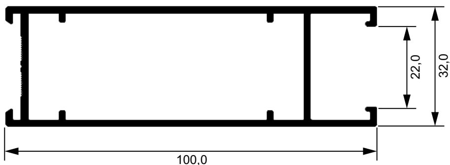
AK511 Marco lateral 5,22 Kg/Br Linha Aglo 2.0
