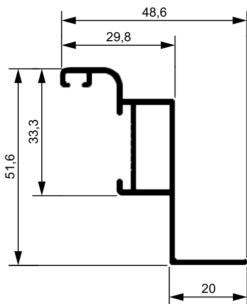
SK046 Marco com arremate 2,88 Kg/Br
