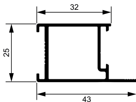
90120 Montante da folha 2,87 Kg/Br
