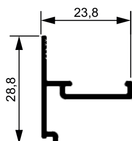
SK292 Inversor de baguete. 1,26 Kg/Br
