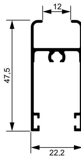
90186 Travessa superior 3,07 Kg/Br e inferior
