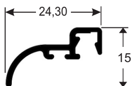
LO091 Pingadeira maximar 0,95 Kg/Br
