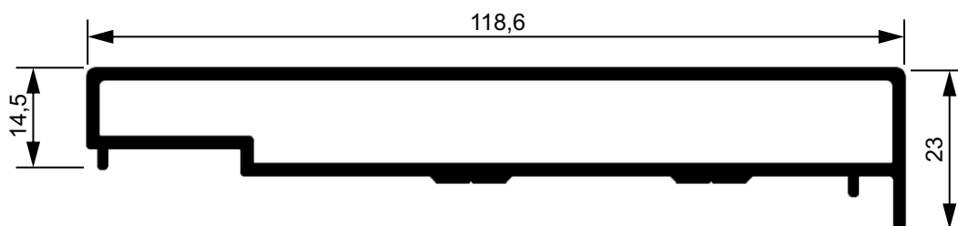
NG100 Perfil superior retangular para corrimão Neograd 7,38 Kg/Br
