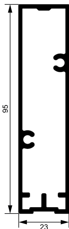
NG102 Montante para corrimão Neograd 7,12 Kg/Br
