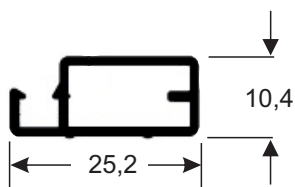
TR163 Perfil tela mosquiteiro para janela leve 1,25 Kg/Br
