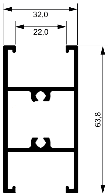
AK510 Travessa intermediária 5,70 Kg/Br Linha Aglo 3.2
