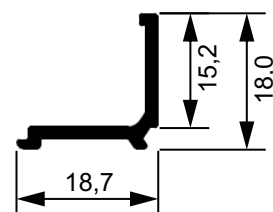
AK418 Baguete 0,89 Kg/Br
