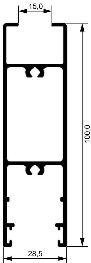
AK303 Travessa inferior e superior. 7,46 Kg/Br Linha Aglo 3.2
