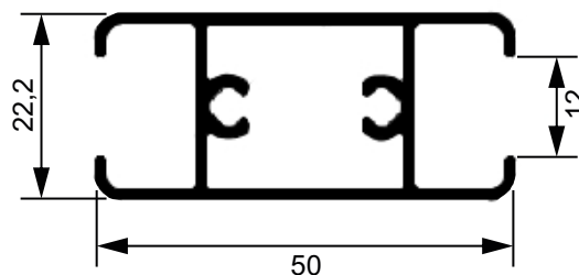
SK118 Travessa central da folha 3,59 Kg/Br
