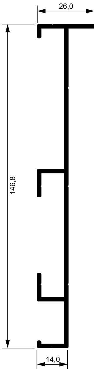
AK505 Marco lateral 3 planos 6,13 Kg/Br Linha Aglo 3.2
