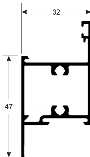
LO076 Travessa maxim-ar para peitoril 5,05 Kg/Br
