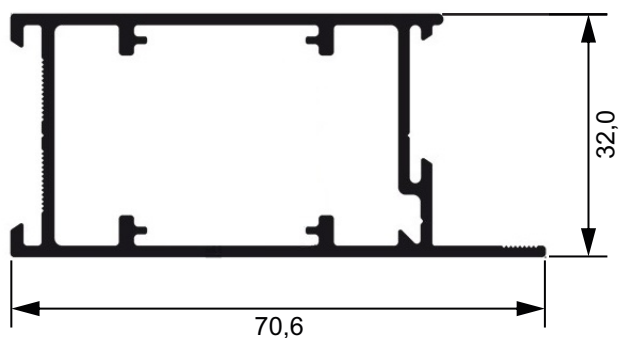
AK356 Travessa intermediária 4,53 Kg/Br Linha Aglo 3.2
