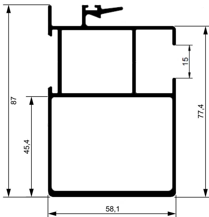
AK309 Montante mão amiga com reforço tubular. Linha Aglo 3.2 10.29 Kg/Br
